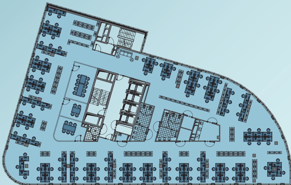
PIĘTRA 2-7, ARANŻACJA OPEN SPACE FLOORS 2-7, OPEN SPACE ARRANGEMENT SOLUTION
